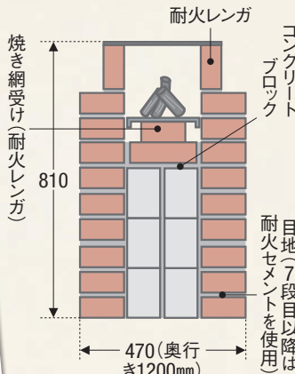
BBQ炉断面図
